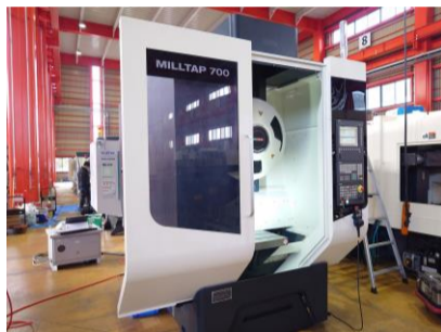
タッピングセンター 森精機 MILLTAP700 2015年製 SINUMERIK BBT30 管理番号:P008396 置場:東日本マシンプラザ
