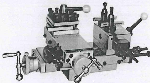
●ネジ送り刃物台
